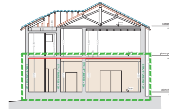
SEZIONE A-A
